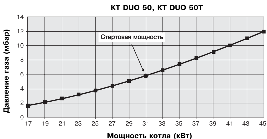
График настройки теплопроизводительности аппарата
